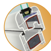
Système à 5 chambres ouvrant semi-en décalé
