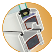
Système 5 chambres ouvrant en en décalé
